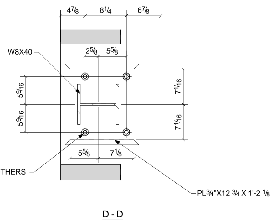
D - D
