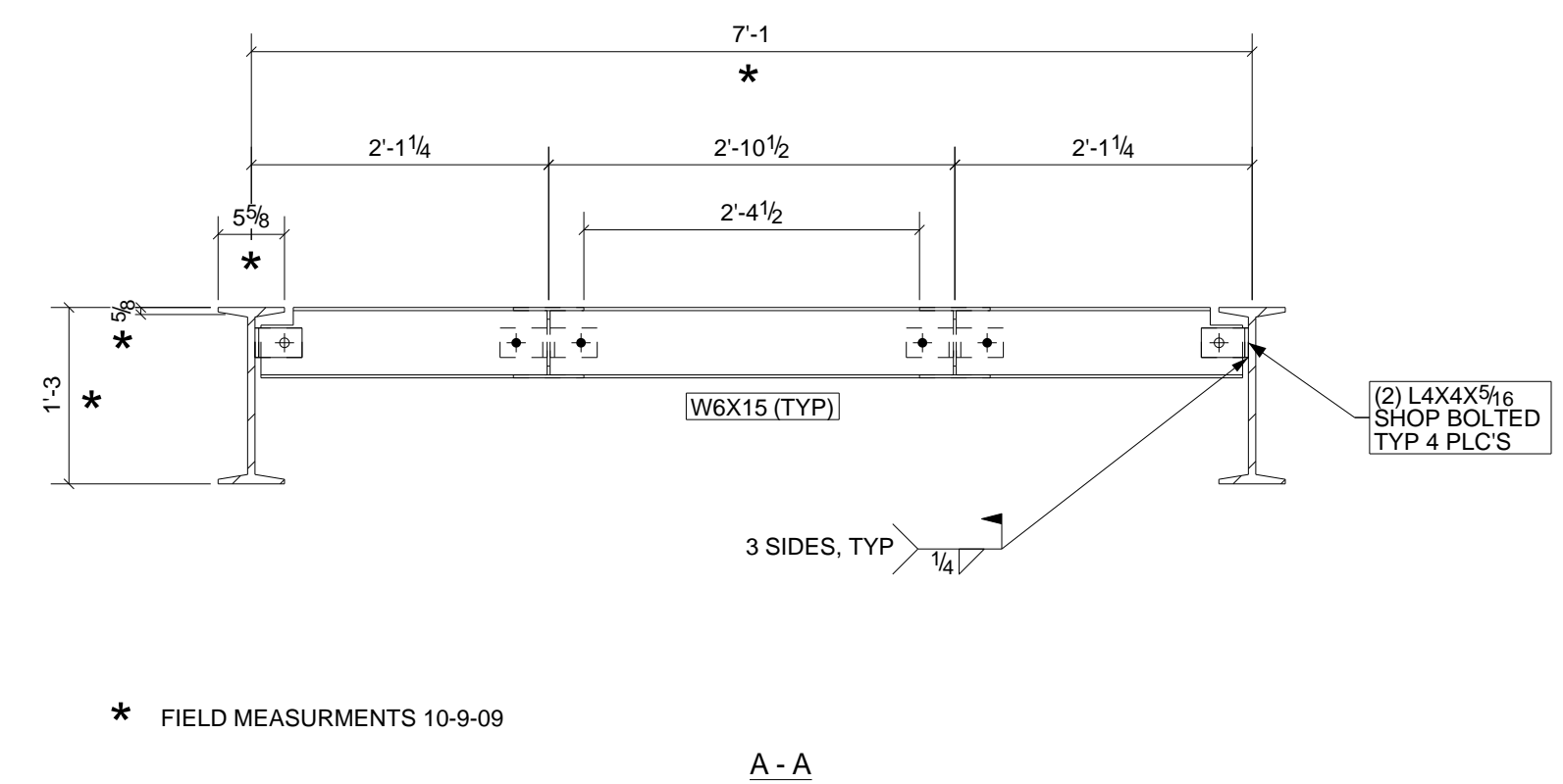
A - A
